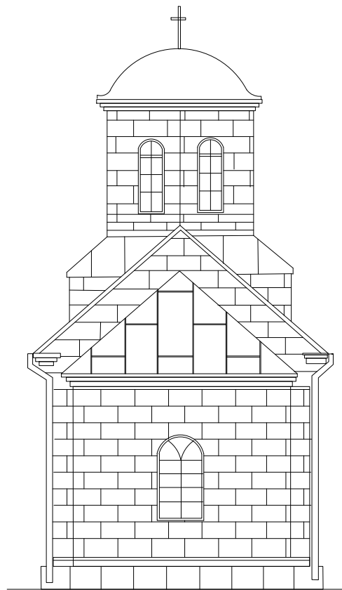
ISTOČNA FASADA
